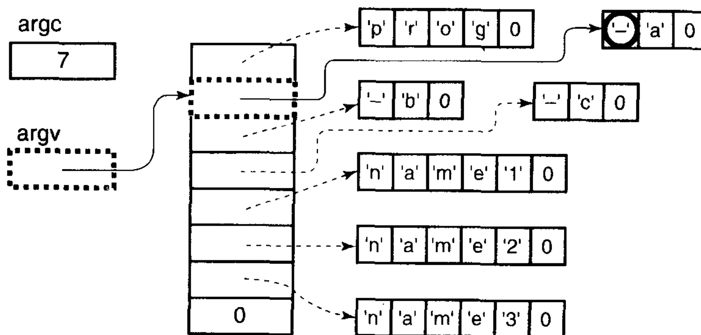
图 13.2 访问参数
