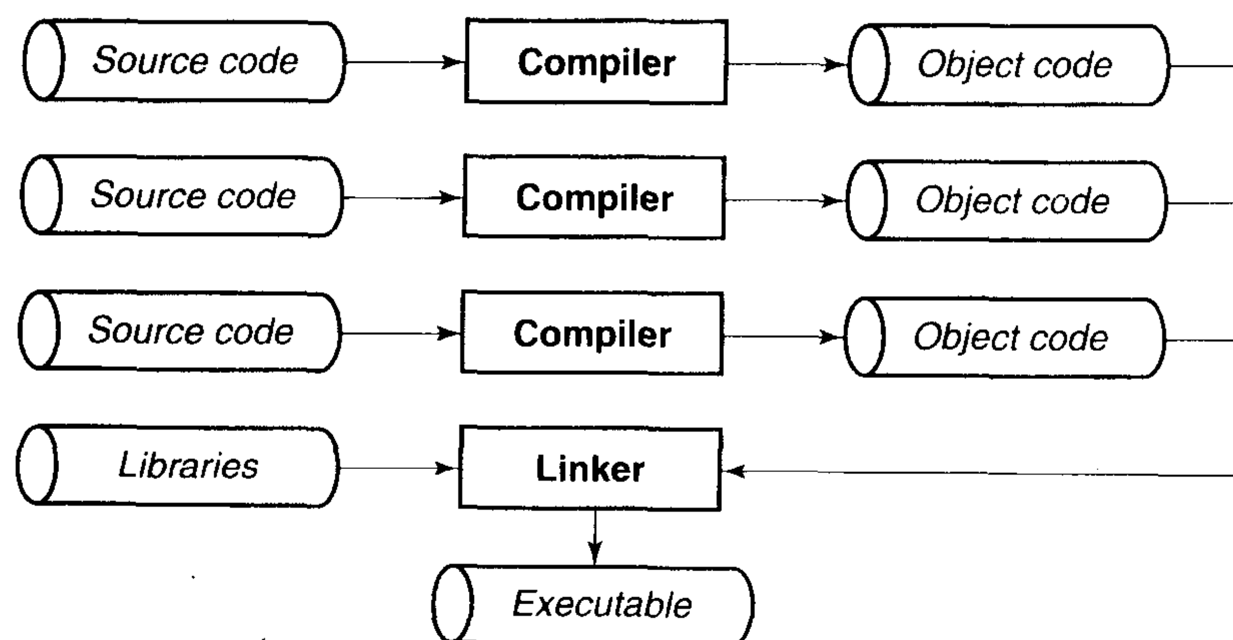
图 2.1 编译过程
